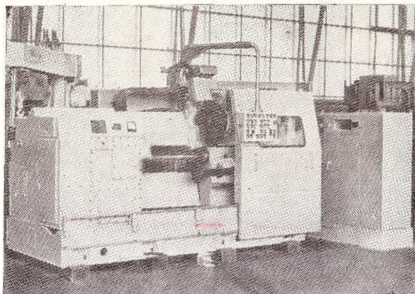
Токарный полуавтомат с числовым программным управлением мод. 1Б732ФЗ
